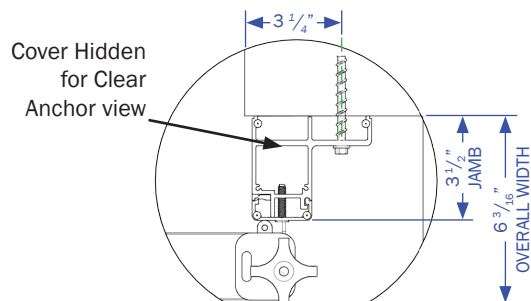
JAMB DETAIL
