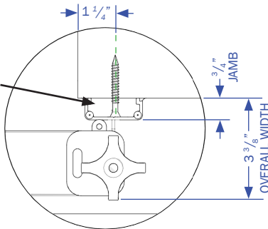
JAMB DETAIL
